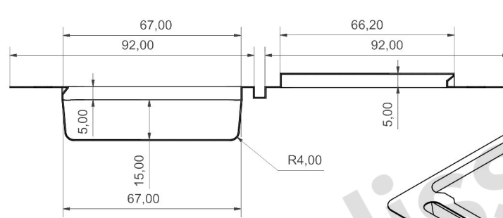
A-A (1:1)
