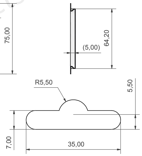
C-C (0,70 : 1)
