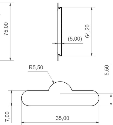
C-C (0,70 : 1)
