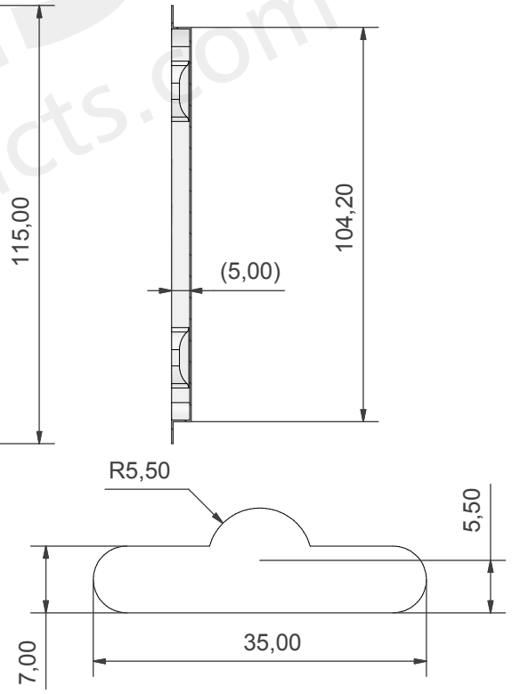
C-C (0,80 : 1)
