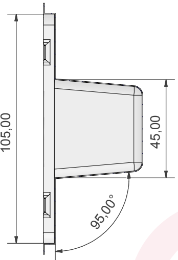
B-B (0,80 : 1)
