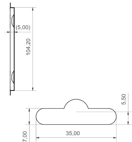
C-C (0,70 : 1)
