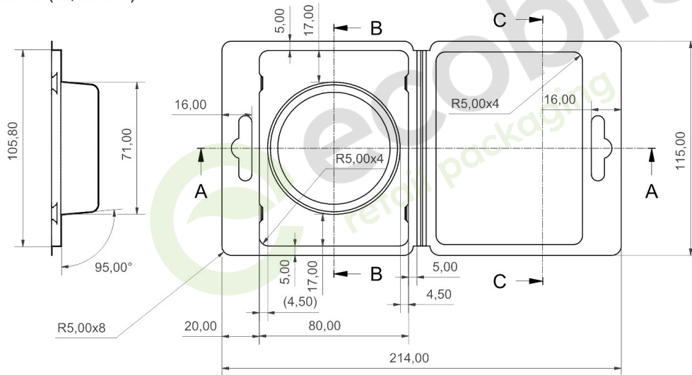
B-B (0,70 : 1)
