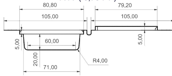
A-A (0,70 : 1)
