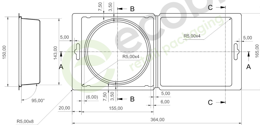
B-B (1:2)
