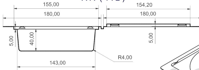
A-A (1:2)
