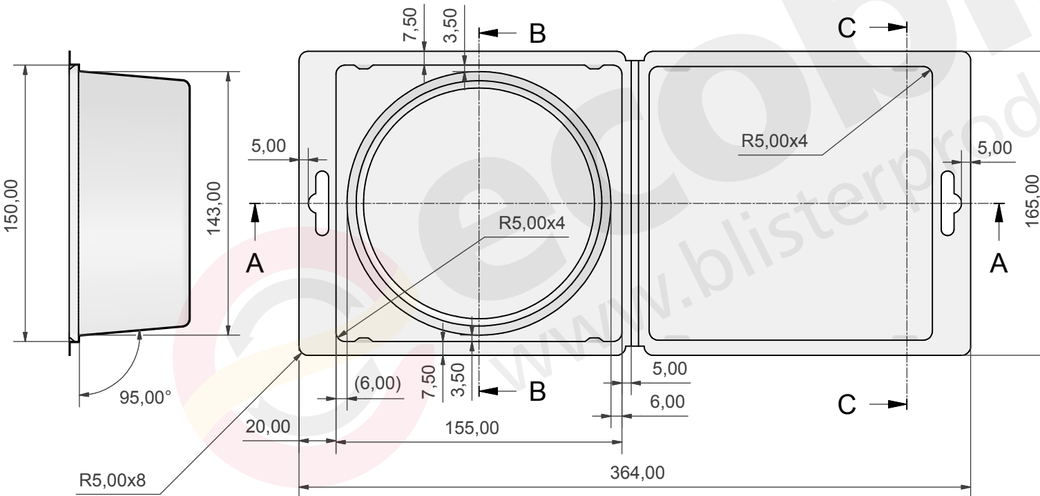
B-B (1:2)
