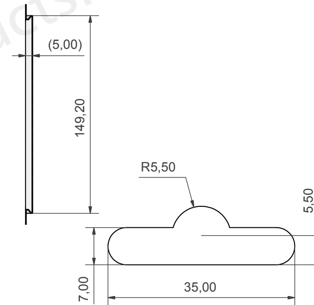
C-C (1:2)
