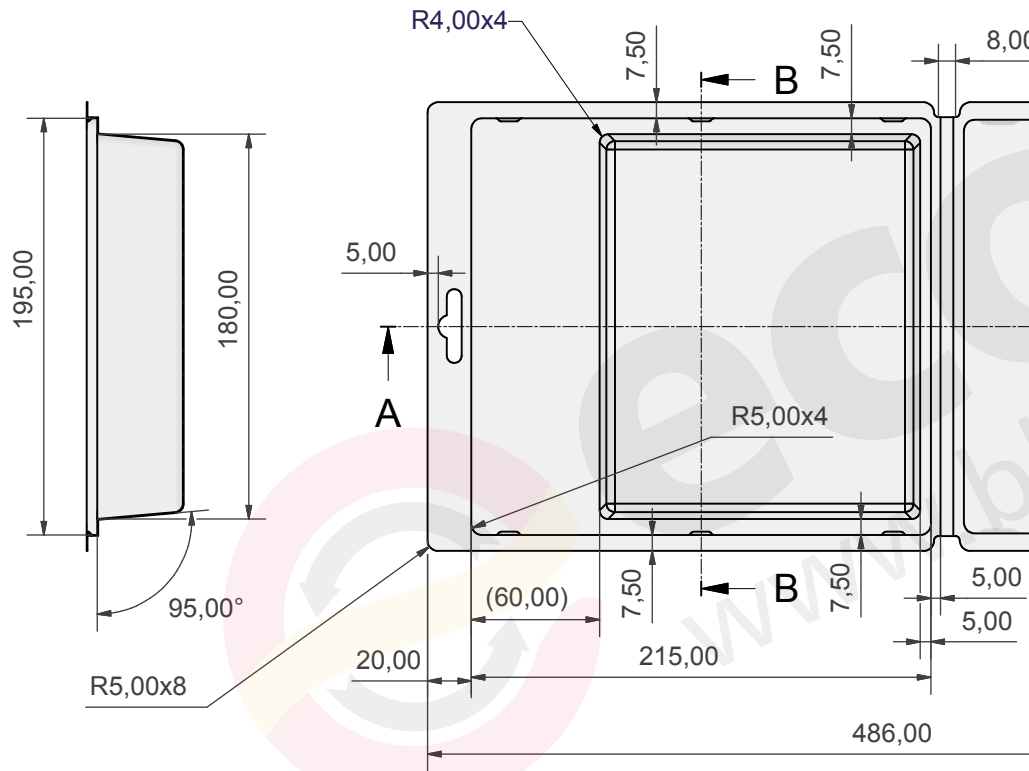
B-B (0,40 : 1)
