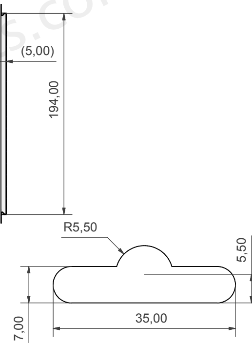
C-C (0,40 : 1)
