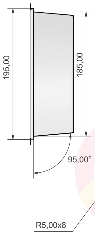
B-B (0,40 : 1)
