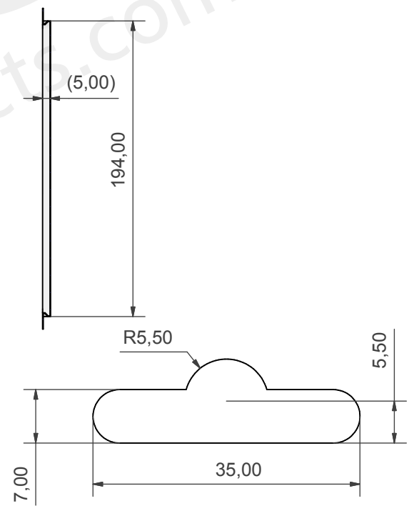
C-C (0,40 : 1)
