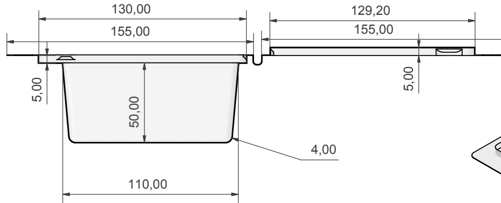
A-A (0,60 : 1)
