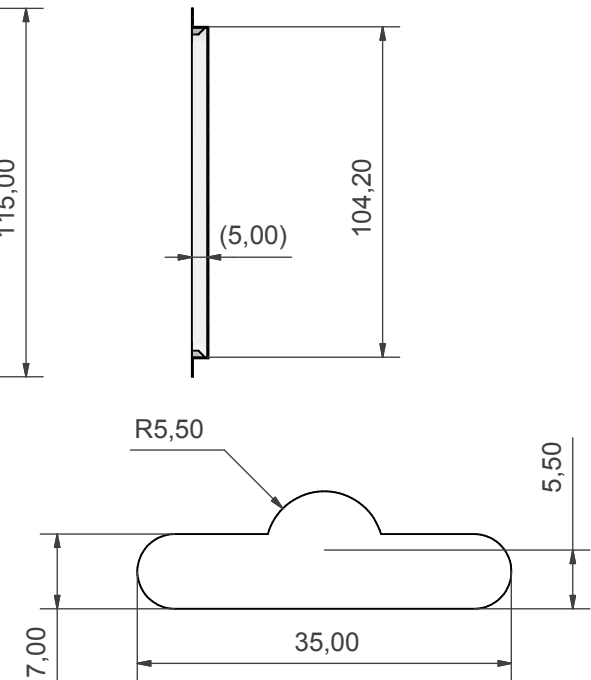
C-C (0,60 : 1)
